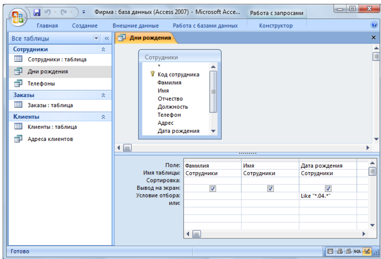
Рис. 5. Создание запроса
