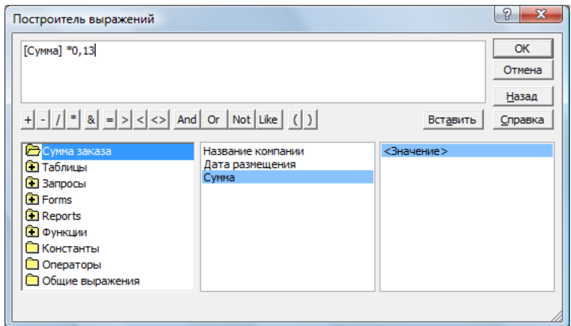
Рис. 8. Построитель выражений
