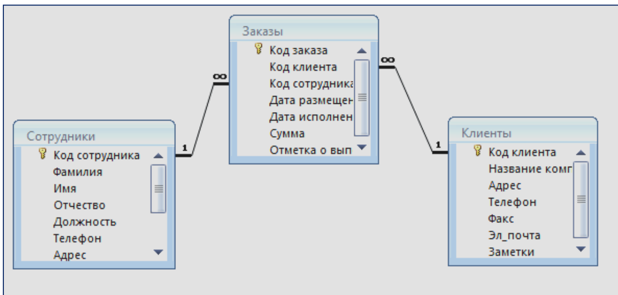
Рис. 2. Схема данных
