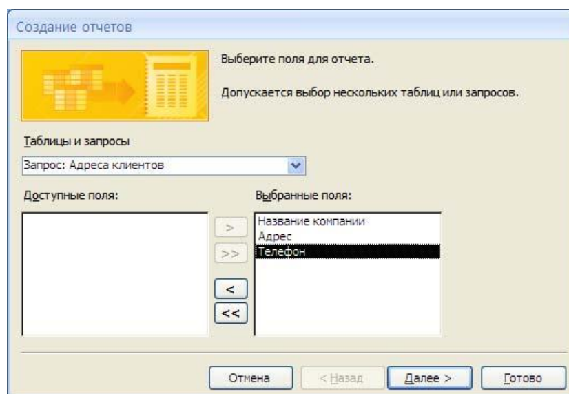
Рис. 15. Мастер отчетов
